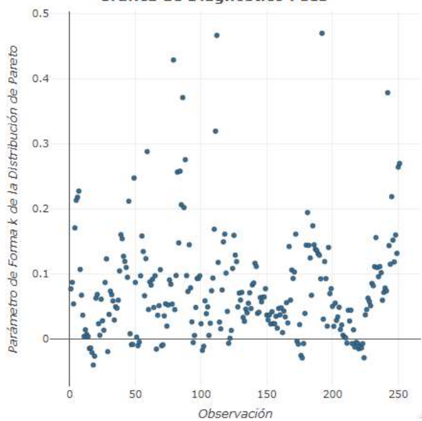
Figura 4 Diagnóstico de Muestreo de Importancia Suavizado por Pareto (PSIS) Gráfica de Diagnóstico PSIS
