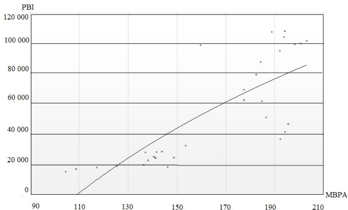
Figura 4. Modelo logarítmico.
