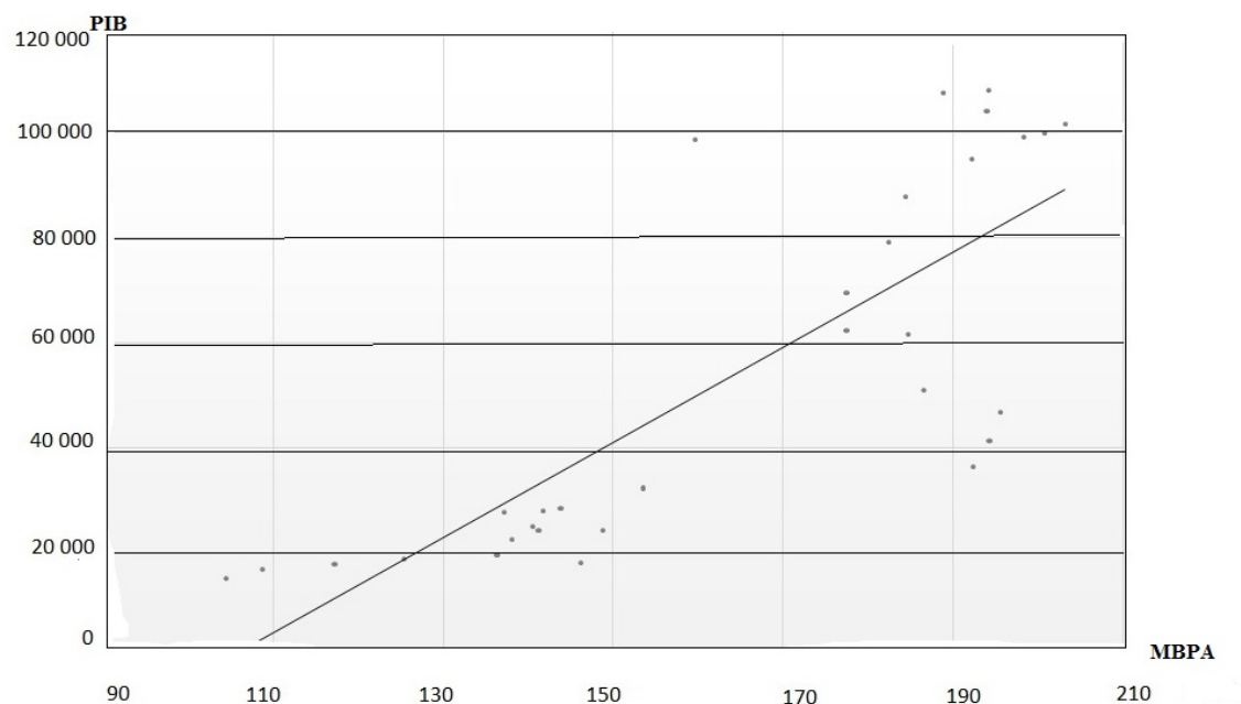
Figura 3. Regresión lineal.
