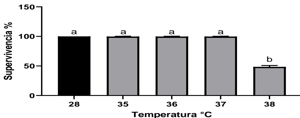
Figura 1. Determinación de una NLHS temperatura en camarones P. vannamei . La barra T corresponde al valor del ES, letras diferentes denotan diferencias significativas ( p < 0,05 ) entre los grupos según HSD Tukey).
