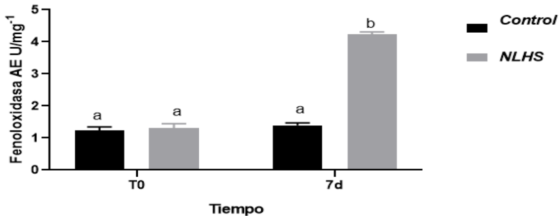
Figura 3. Actividad enzimática específica de Fenoxidasa en camarones P. vannamei expuesto a un NLHS crónico. Los datos representan las medias y el ES (barras T); letras diferentes representan diferencias significativas entre los grupos ( P < 0,05 ) según t de Student.
