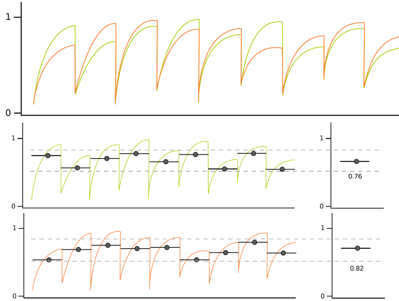
Figura 2: Rendimiento de dos algoritmos sobre un POD. La cuestión que se plantea es ¿cuál es mejor?
