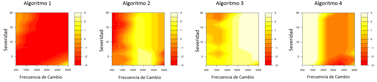
Figura 3: Resultados obtenidos mediante la técnica SRCS. Dado un algoritmo, se construye un ranking que indica, en cada escenario, a cuantos algoritmos “le gana” y con cuantos “pierde”. Este ranking se transforma en una escala de color. Colores más claros indican que el algoritmo en cuestión es mejor que los otros en el escenario considerado.
