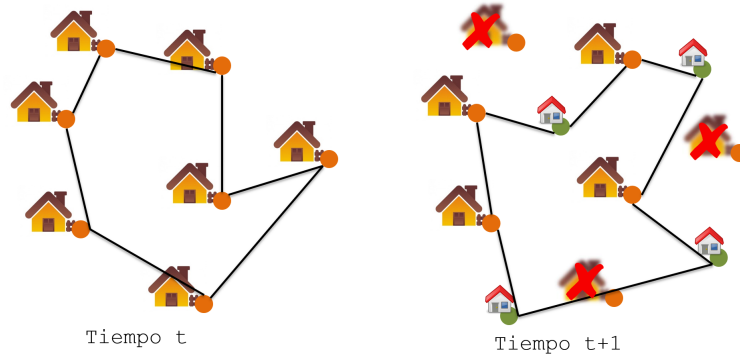
Figura 1: Ejemplo del problema del viajante dinámico: las ciudades pueden aparecer y desaparecer.
