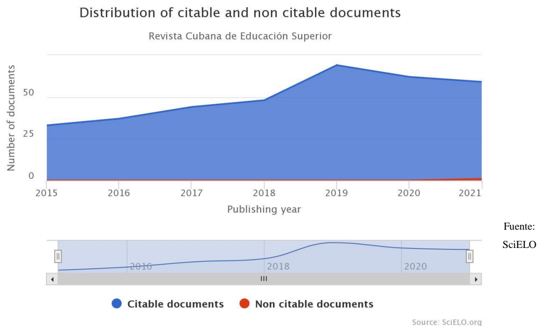
Figura 1. Distribución de documentos citables y no citables (2015-2021).
