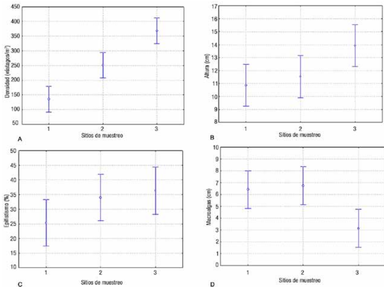
Fig. 2. Estado de la densidad (A), altura de la canopia (B), porcentaje de epifitismo (C) y porcentaje de macroalgas (D) en los pastos marinos de cayo Paredón Grande. 1 y 2: sitios donde no debe existir una acción directa del hombre y 3: sitio donde habrá futuro desarrollo turístico.
